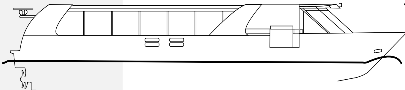
Seitenansicht
